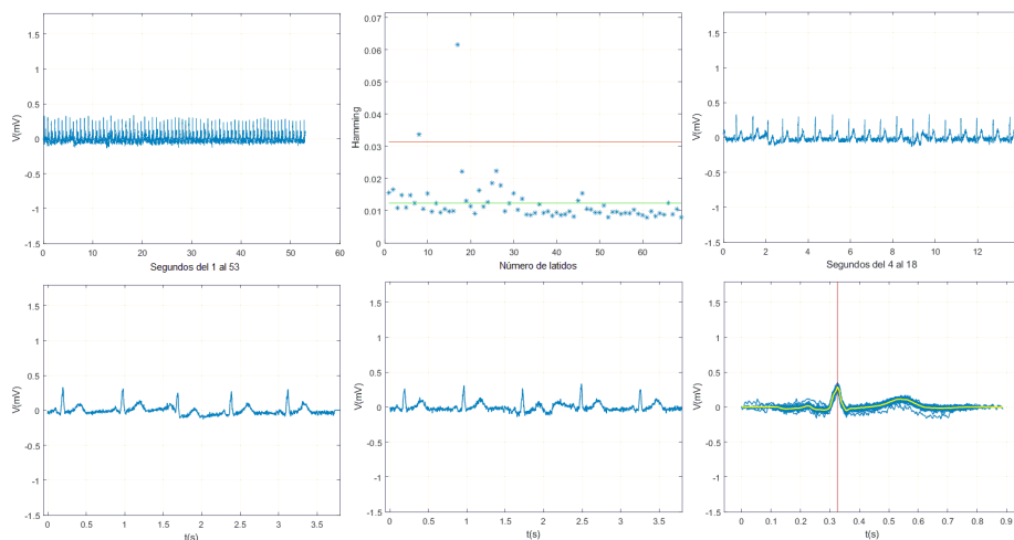
Figura 3. Presentación de los resultados de análisis de un ECG normal usando el sistema 'asistente', derivada I
